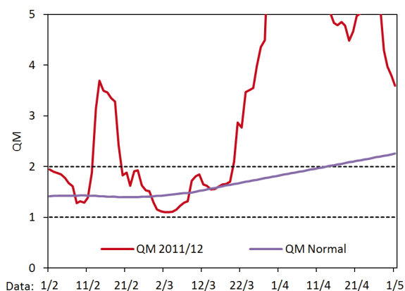
Fig. 3. Temperatura, chuva, insolação, dias de chuva e balanço hídrico de cultivo (CAD = 60 mm) e Quociente Heliopluiométrico de Maturação (QM), em Vacaria, RS, safra 2011/2012. Fonte dos dados: INMET e Embrapa Uva e Vinho. Abreviações e legenda: Mínima abs: mínima absoluta; Máxima abs: máxima absoluta; Média mín: média das mínimas; Média máx: média das máximas; Insol.: insolação; D. chuva: dias do mês com chuva; ARM: armazenamento hídrico; DEF: deficiência hídrica; EXC: excedente hídrico.
