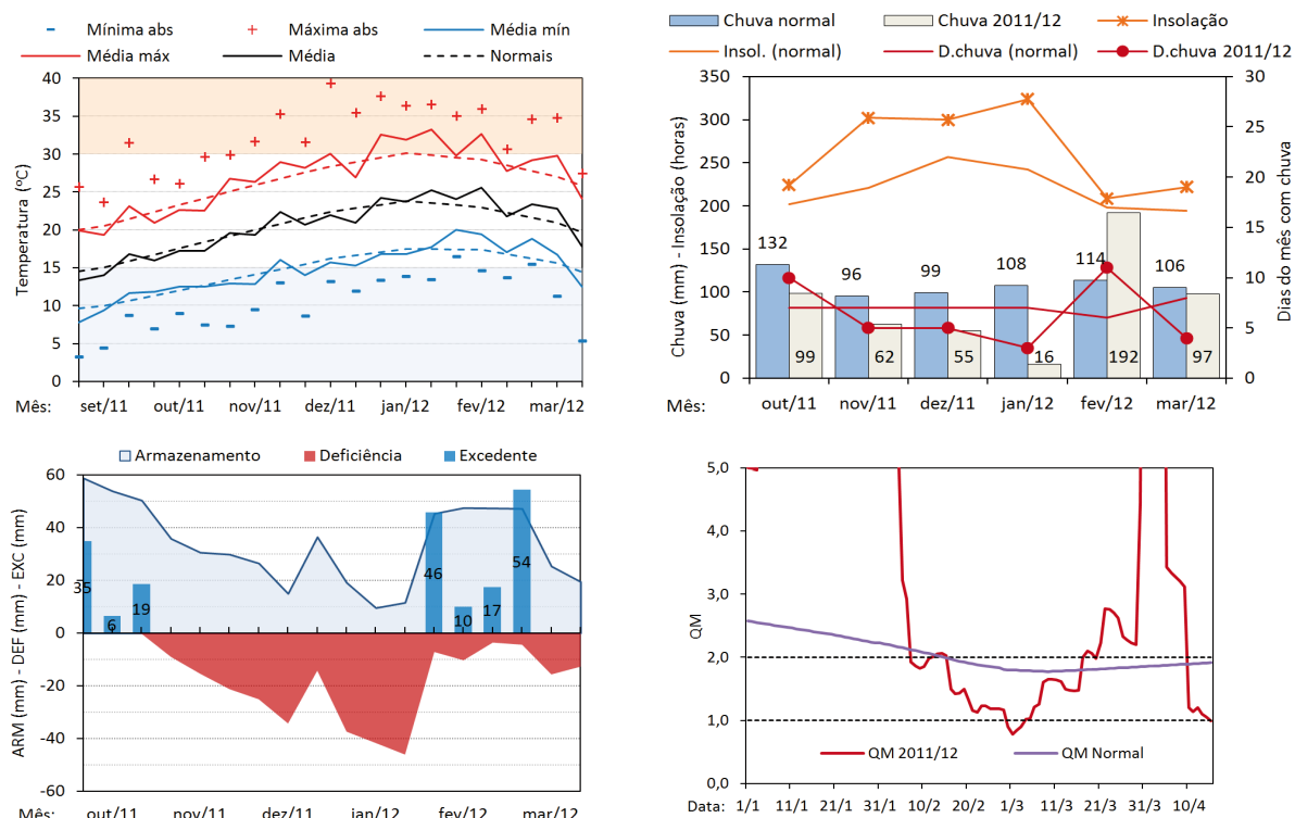
Fig. 6. Temperatura, chuva, insolação, dias de chuva e balanço hídrico de cultivo (CAD=60 mm) e Quociente Heliopluiométrico de Maturação (QM), em Santana do Livramento, RS, safra 2011/2012. Fonte dos dados: INMET. Abreviações e legenda: Mínima abs: mínima absoluta; Máxima abs: máxima absoluta; Média mín: média das mínimas; Média máx: média das máximas; Insol.: insolação; D. chuva: dias do mês com chuva; ARM: armazenamento hídrico; DEF: deficiência hídrica; EXC: excedente hídrico.
