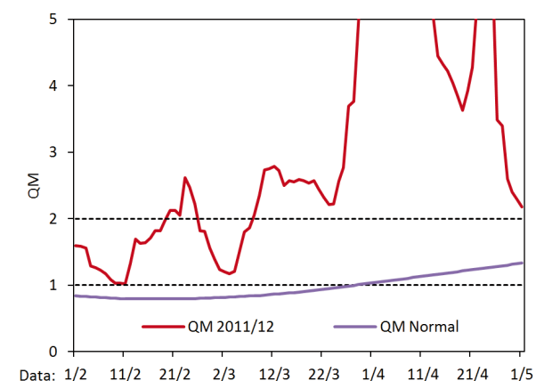
Fig. 2. Temperatura, chuva, insolação, dias de chuva e balanço hídrico de cultivo (CAD=60 mm) e Quociente Heliopluiométrico de Maturação (QM), em São Joaquim, SC, safra 2011/2012. Fonte dos dados: INMET. Abreviações e legenda: Mínima abs: mínima absoluta; Máxima abs: máxima absoluta; Média mín: média das mínimas; Média máx: média das máximas; Insol.: insolação; D. chuva: dias do mês com chuva; ARM: armazenamento hídrico; DEF: deficiência hídrica; EXC: excedente hídrico.
