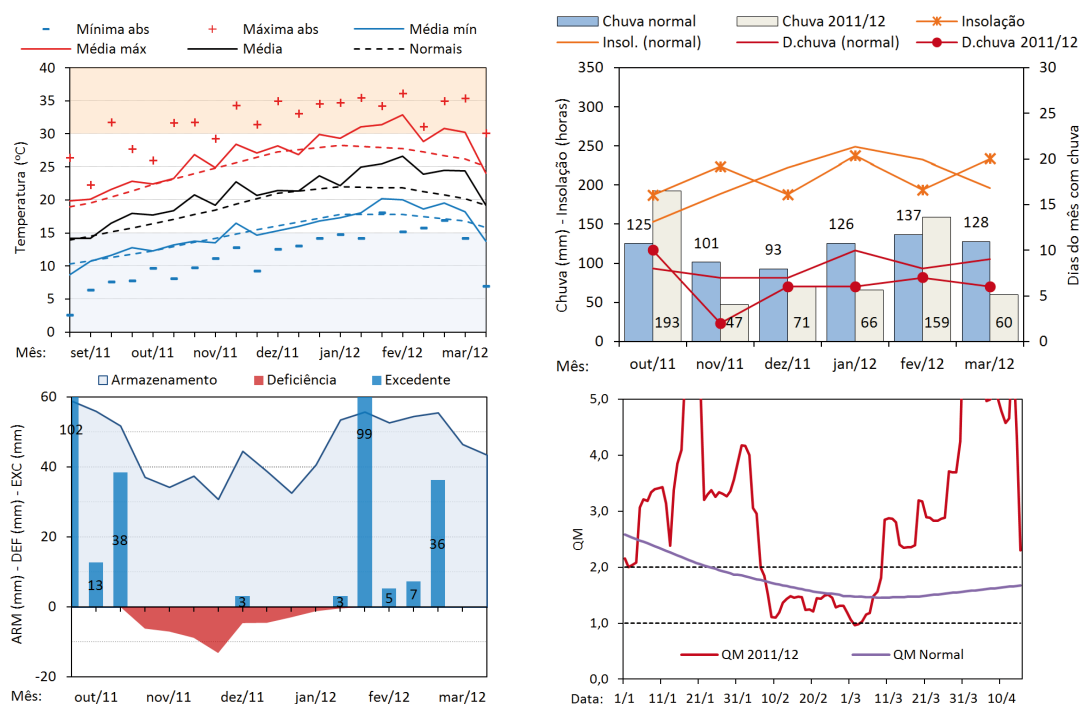
Fig. 5. Temperatura, chuva, insolação, dias de chuva e balanço hídrico de cultivo (CAD = 60 mm) e Quociente Heliopluiométrico de Maturação (QM), em Encruzilhada do Sul, RS, safra 2011/2012. Fonte dos dados: INMET. Abreviações e legenda: Mínima abs: mínima absoluta; Máxima abs: máxima absoluta; Média mín: média das mínimas; Média máx: média das máximas; Insol.: insolação; D. chuva: dias do mês com chuva; ARM: armazenamento hídrico; DEF: deficiência hídrica; EXC: excedente hídrico.
