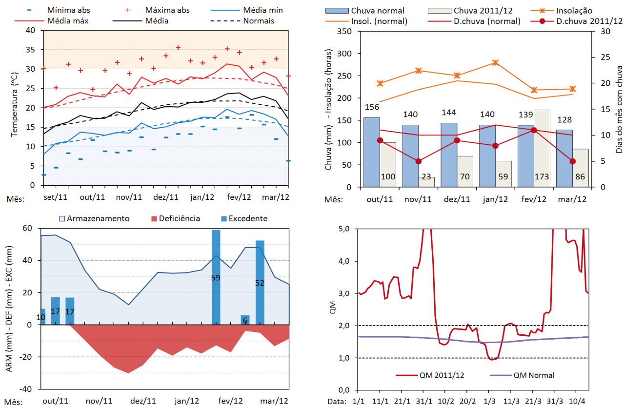
Fig. 4. Temperatura, chuva, insolação, dias de chuva e balanço hídrico de cultivo (CAD = 60 mm) e Quociente Heliopluiométrico de Maturação (QM), em Bento Gonçalves , RS, safra 2011/2012. Fonte dos dados: Embrapa Uva e Vinho. Abreviações e legenda: Mínima abs: mínima absoluta; Máxima abs: máxima absoluta; Média mín: média das mínimas; Média máx: média das máximas; Insol.: insolação; D. chuva: dias do mês com chuva; ARM: armazenamento hídrico; DEF: deficiência hídrica; EXC: excedente hídrico.
